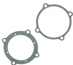
Oliepomp pakking set type-1 motor 25pk, 30pk en 34pk t/m 7.1965, 1200cc t/m 1967 (D 0 230 000), 1300cc t/m 1967 (E 0 013 650 en F 1 225 017), 1500cc t/m 1967 (L 0 018 099 en H 0 822 051), type-3 motor 1500cc t/m 1967 (K 0 090 195), 1600cc t/m 1967 (T 0 445 097)
